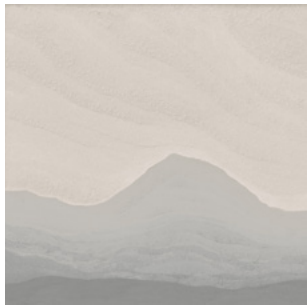
ANDES
