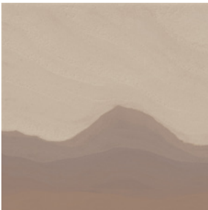
SEDIMENT
