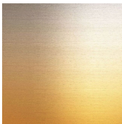
MICA
